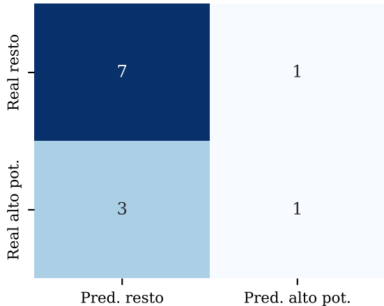
Matriz de confusión (test)
