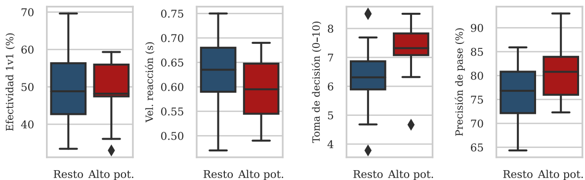
Figura 3: Métricas clave según grupo de potencial.
