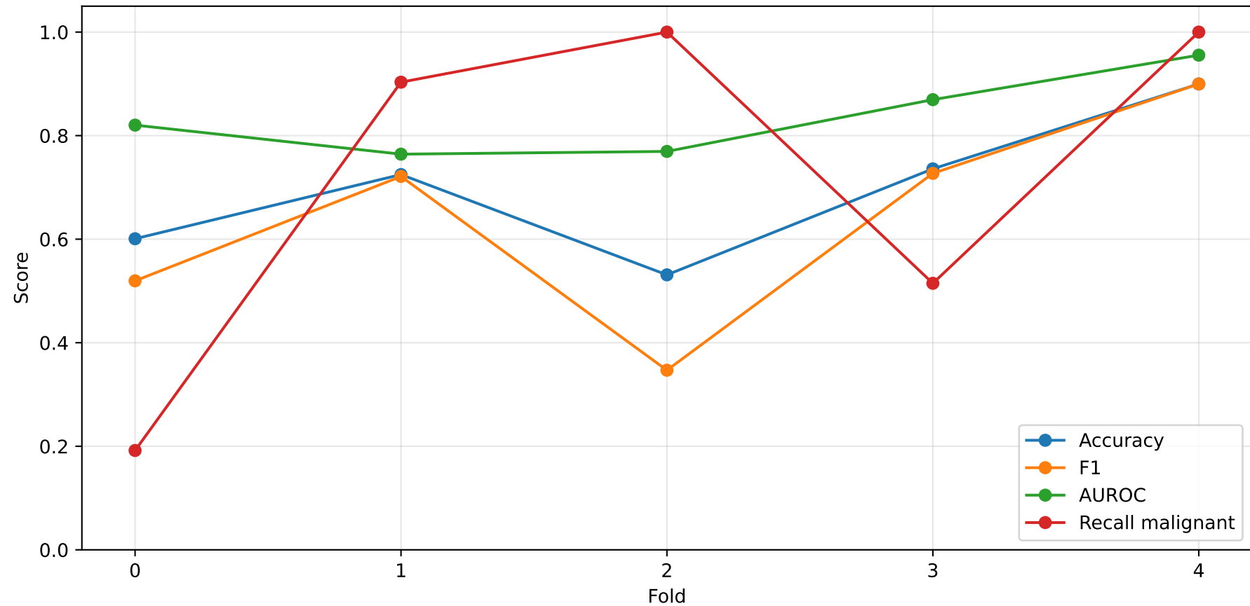
D2 — Variabilità delle metriche sui 5 fold patient-wise
