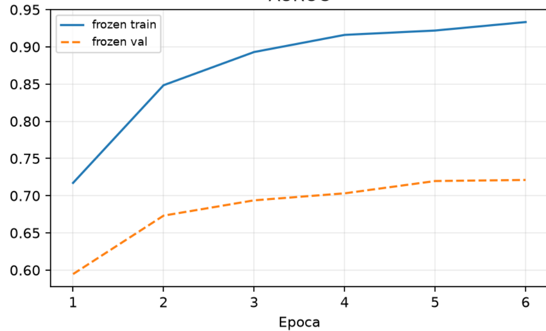
AUROC
