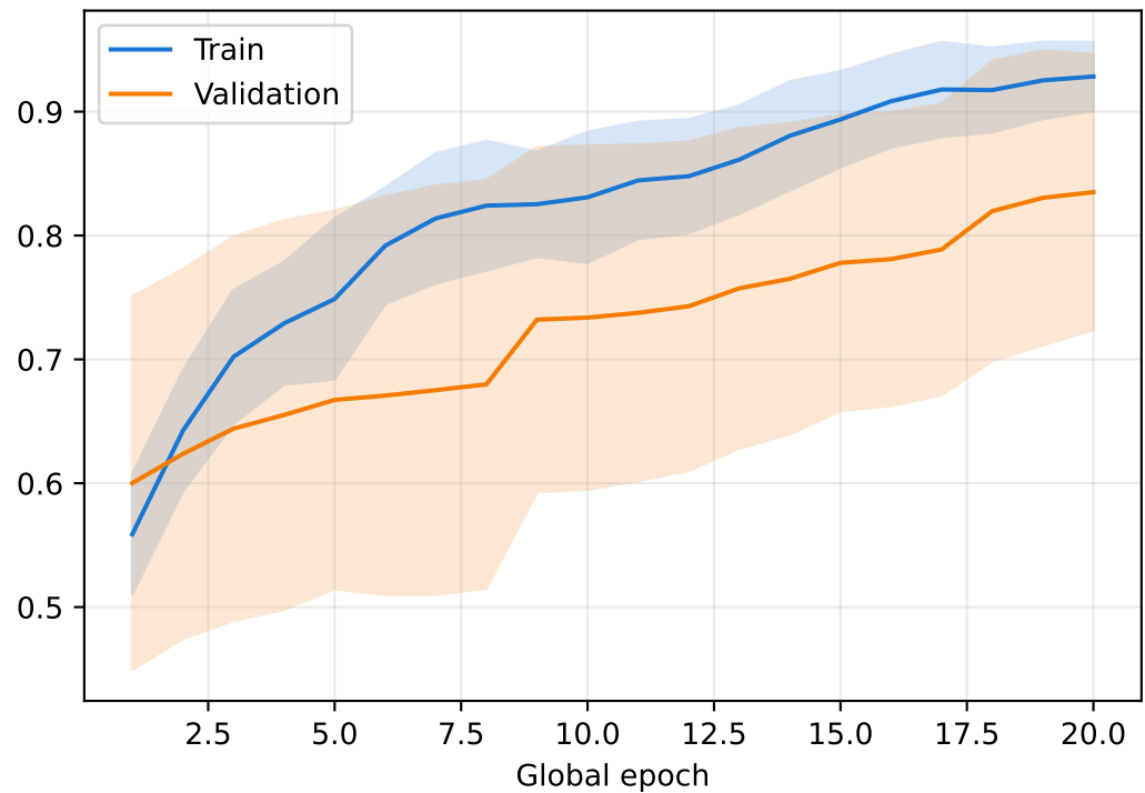
AUROC
