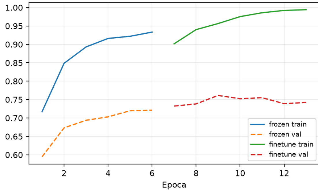
AUROC
