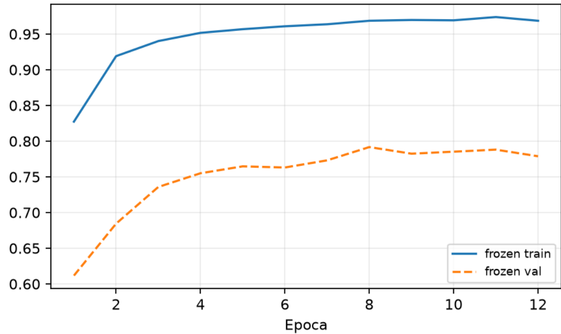
AUROC
