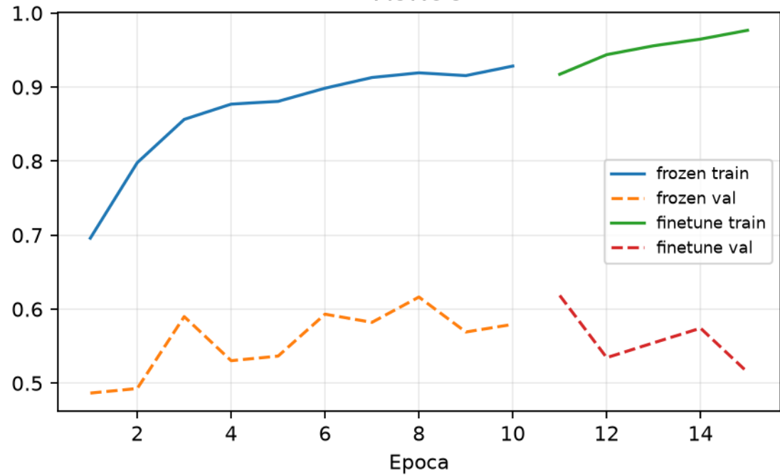
AUROC
