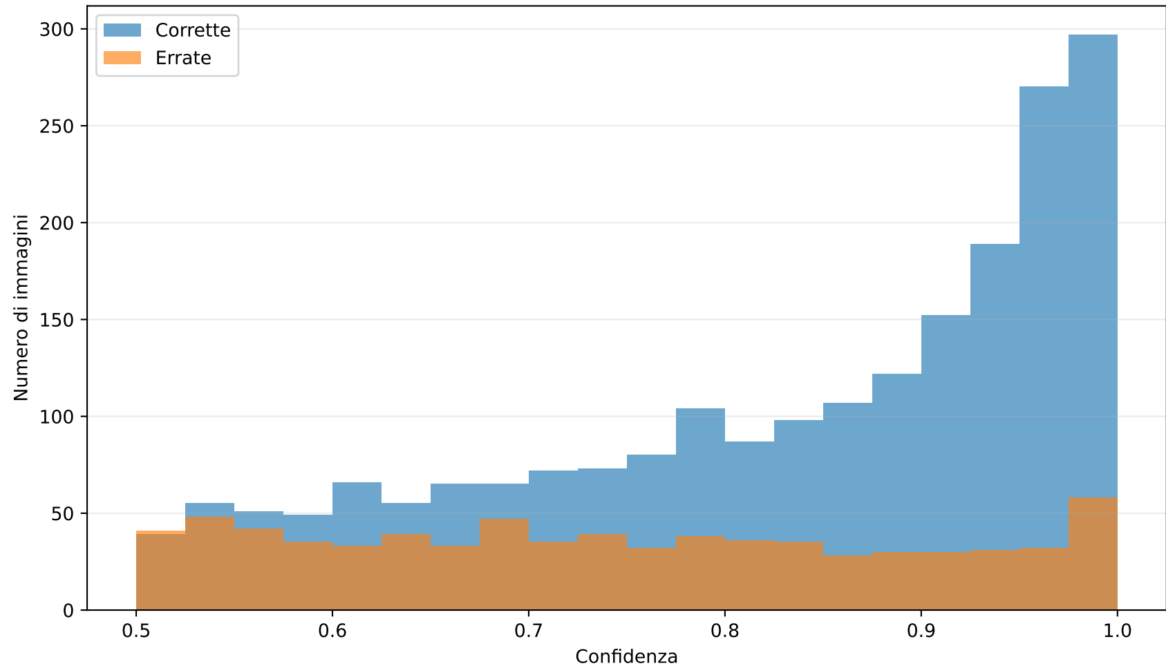
Confidenza: predizioni corrette vs errate
