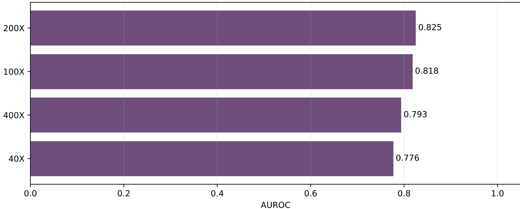
AUROC per ingrandimento — EfficientNetB0 fine-tuned
