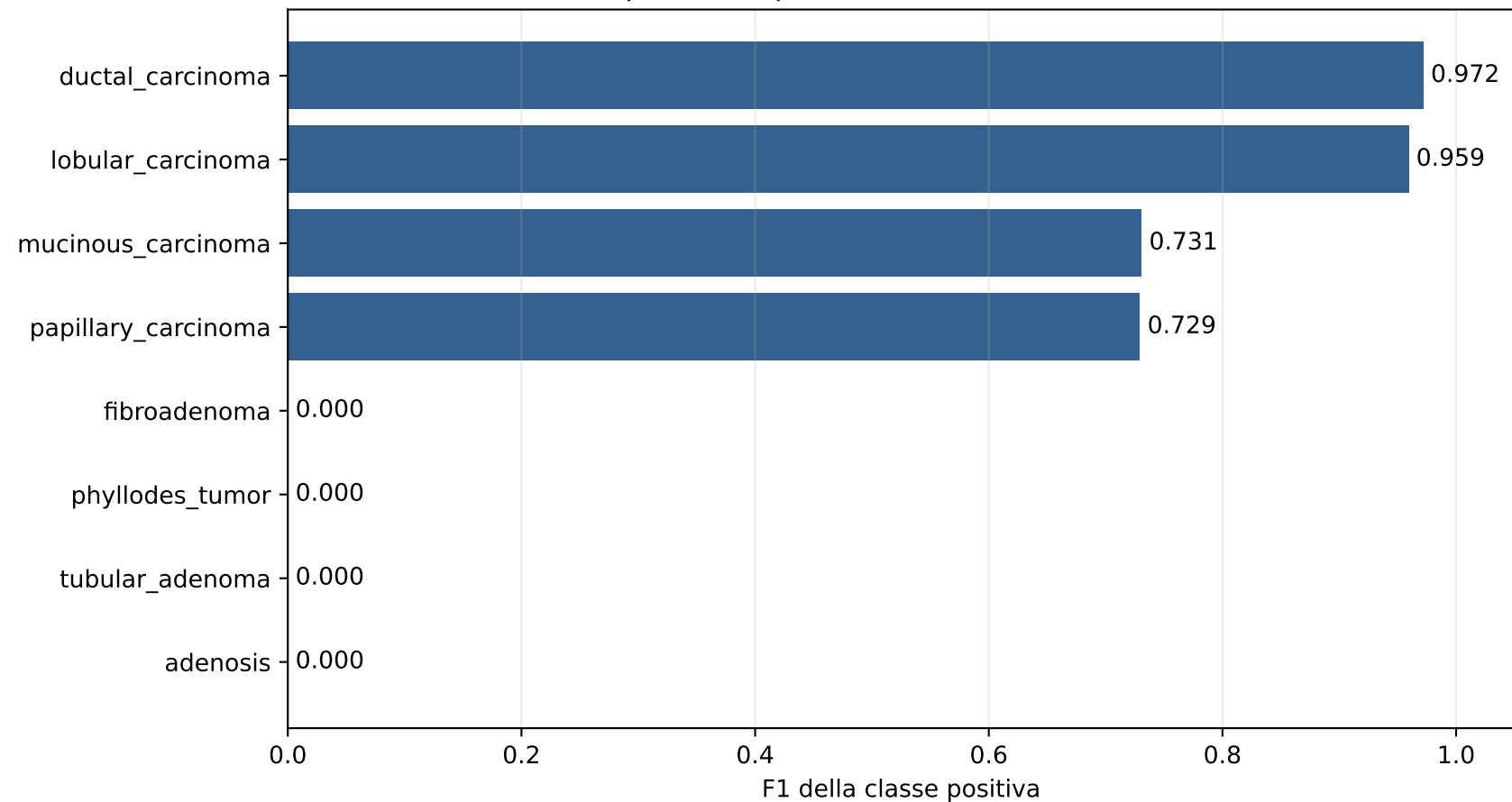
F1 per sottotipo — EfficientNetB0 fine-tuned
