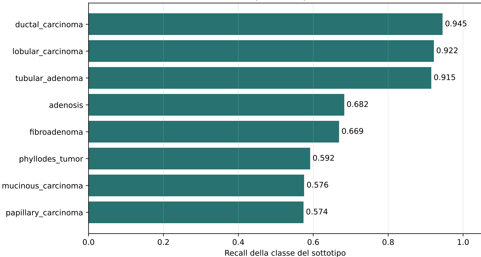
Recall della classe rilevante per sottotipo — EfficientNetB0 fine-tuned
