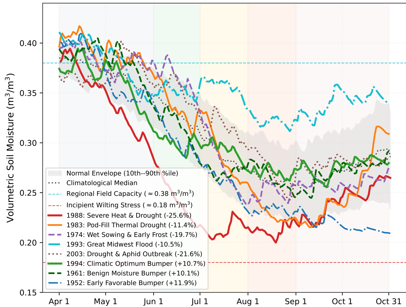
(d) Root-Zone Soil Moisture Depletion (0--100 cm SM_{root} )
