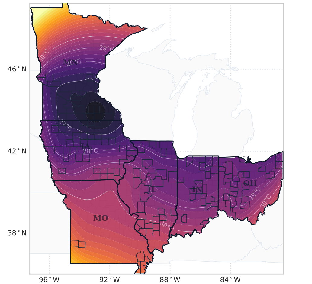
(d) 2016 Climatic Optimum: July-August Max Temp ( T_{\max} )
