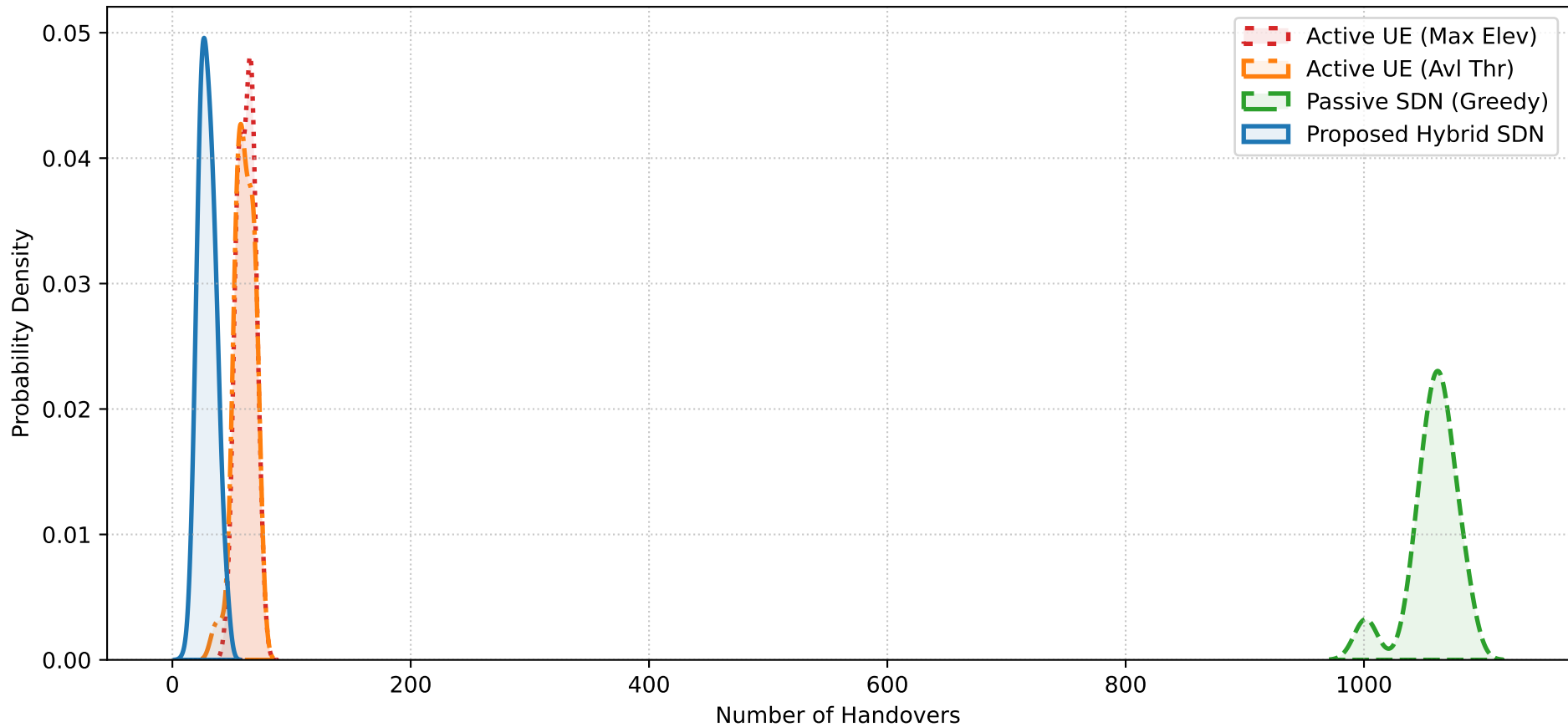
PDF of Intra-Satellite Handovers per UE
