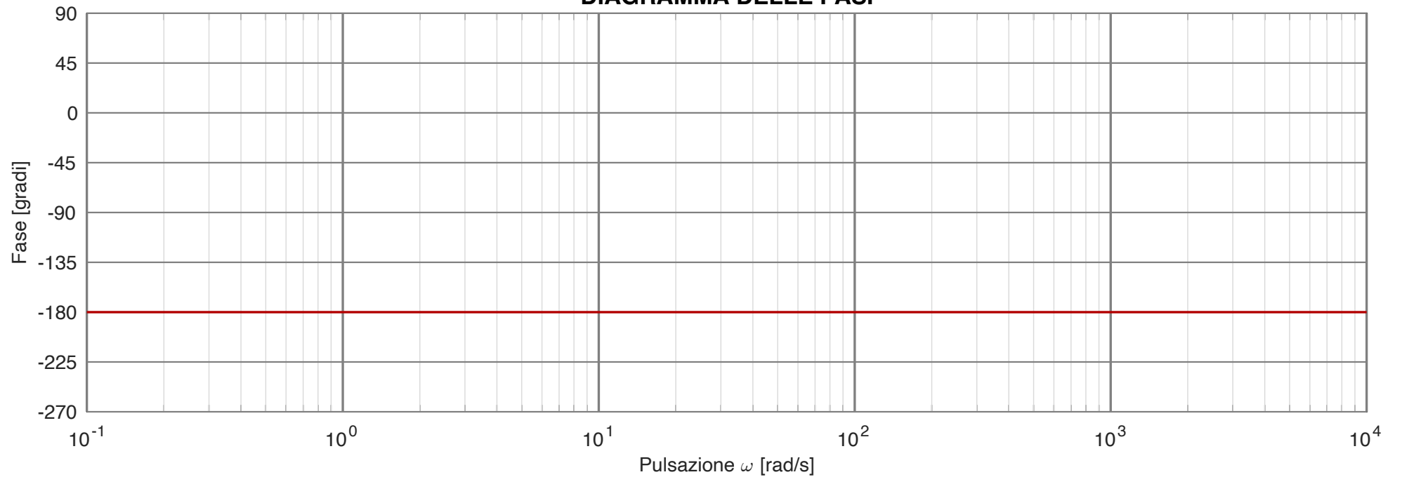
DIAGRAMMA DELLE FASI
