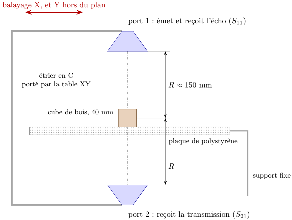
FIGURE 1 – Configuration retenue, vue de côté. Les deux antennes, solidaires, balayent ensemble ; le cube reste fixe sur une plaque de polystyrène ( \varepsilon_r \simeq 1,02 ) tenue hors de la zone balayée.
