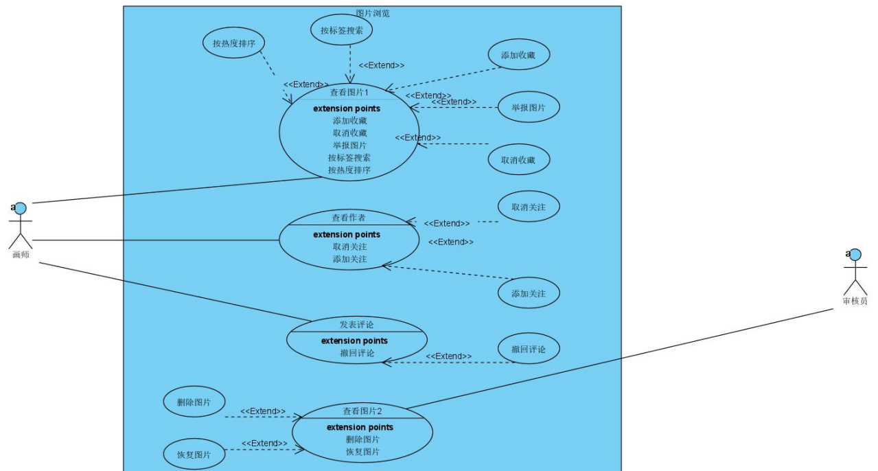
图 3.4 图片浏览用例图
