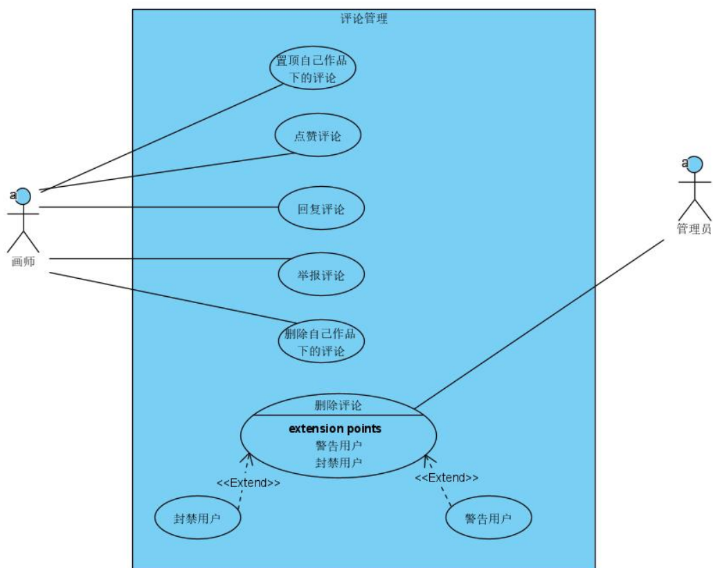
3.5 评论管理用例图
