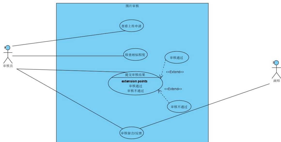
图 3.2 图片审核用例图
