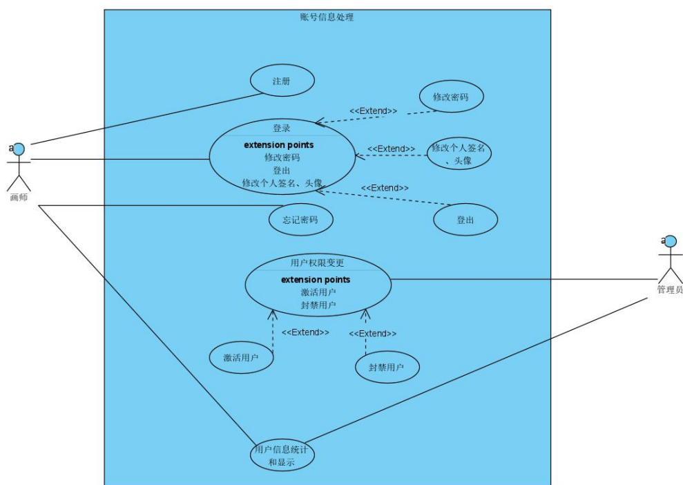
3.6 账号信息处理用例图
