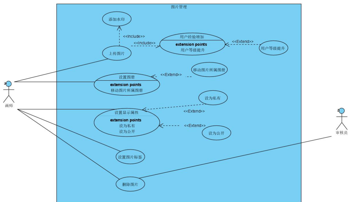
图 3.3 图片管理用例图
