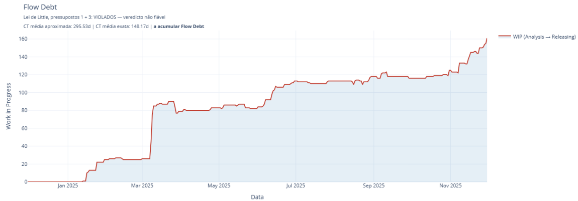
Fig. 11: Flow Debt — evolucao do WIP na janela de avaliacao. O exemplo mostra de proposito um conjunto de dados em que a lei de Little nao se aplica: o WIP cresce sempre, por isso o cabecalho diz „verdict not dependable”.
