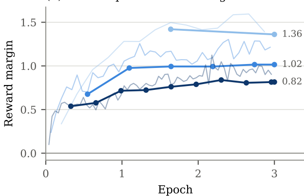
(d) DPO: implicit reward margin
