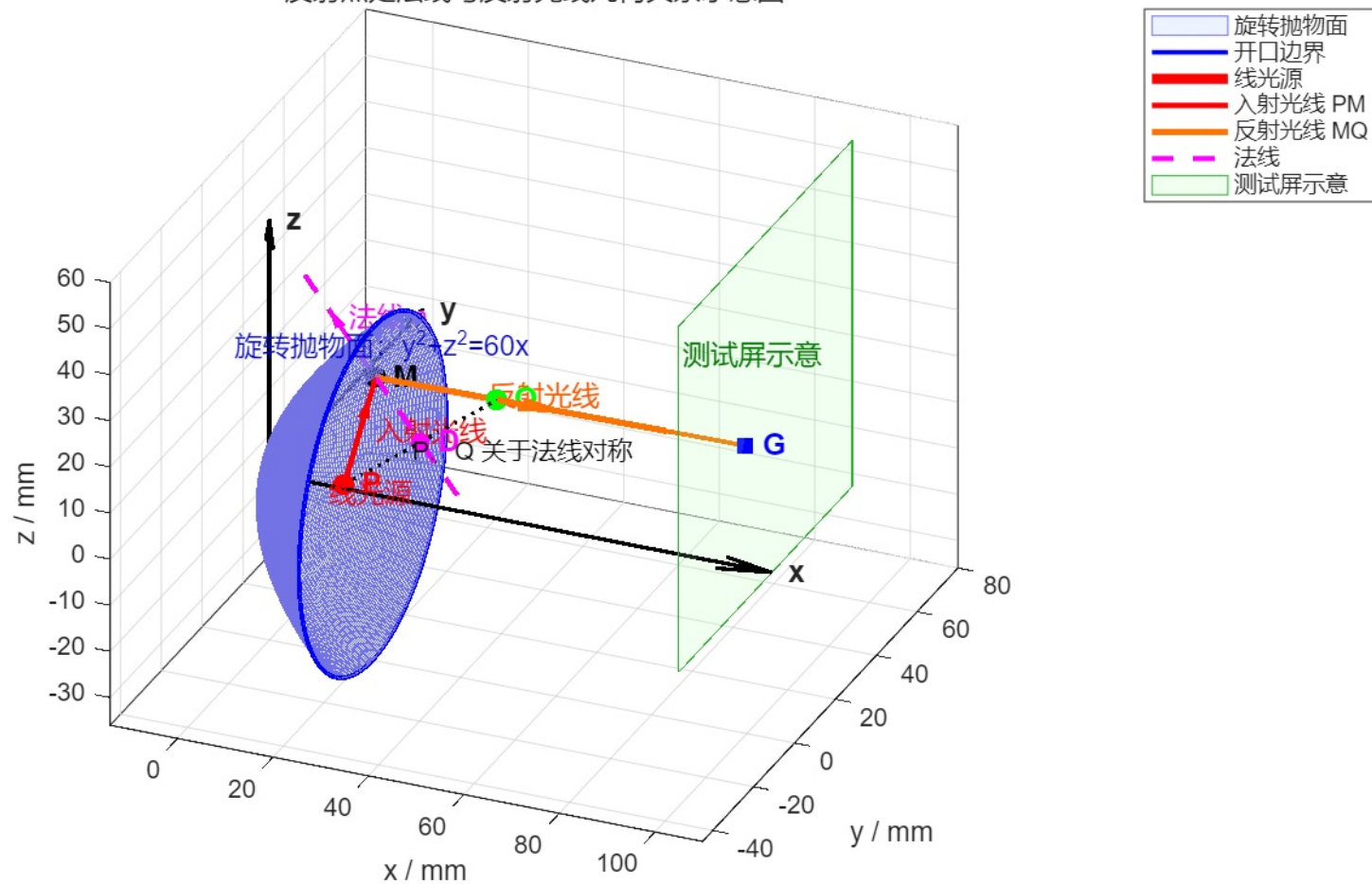
反射点处法线与反射光线几何关系示意图
