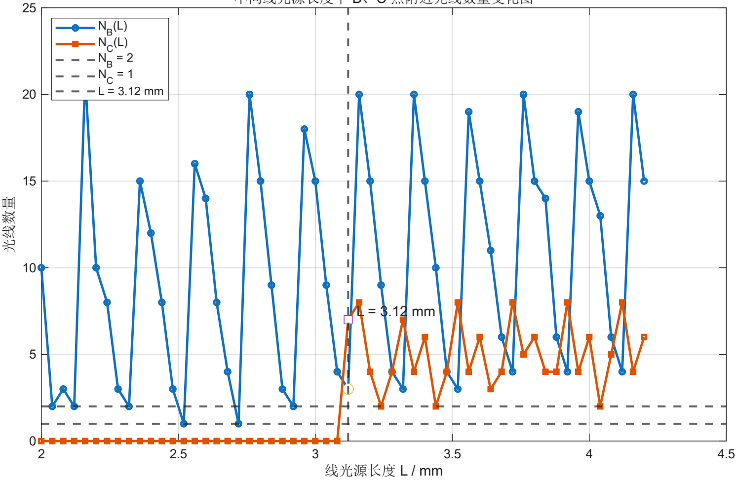
不同线光源长度下 B、C 点附近光线数量变化图
