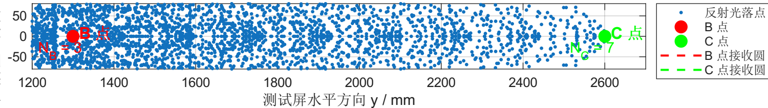
线光源长度 L = 3.12 mm 时测试屏上 B、C 点附近落点分布图
