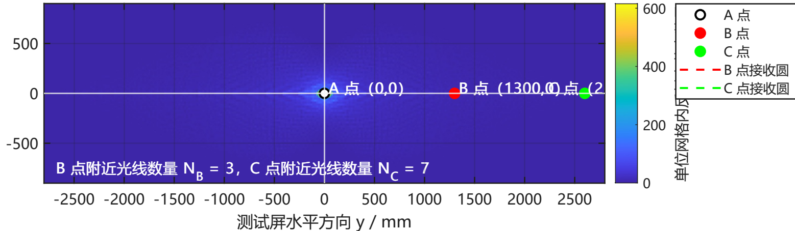
线光源长度为 3.12mm 时测试屏反射光亮区密度分布图
