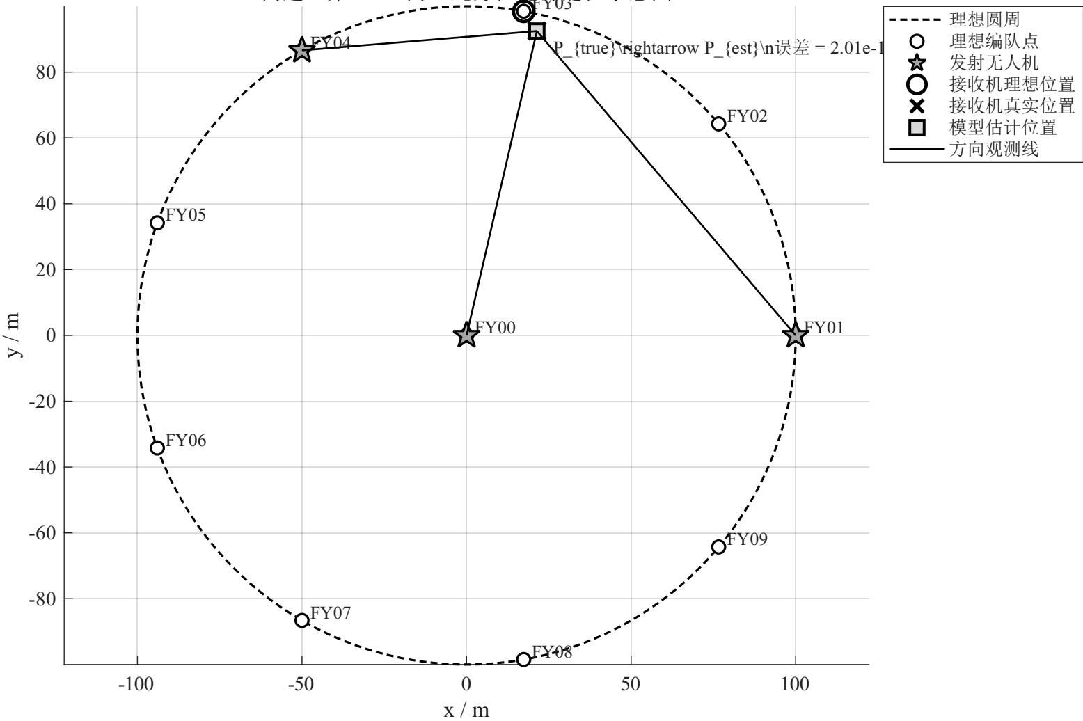
问题一第 (1) 问：纯方位无源定位示意图
