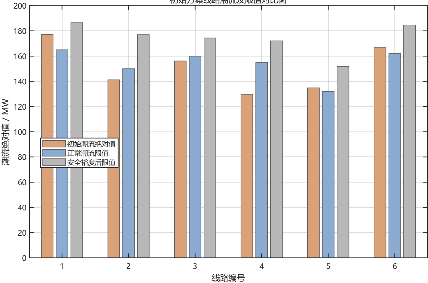
初始方案线路潮流及限值对比图
