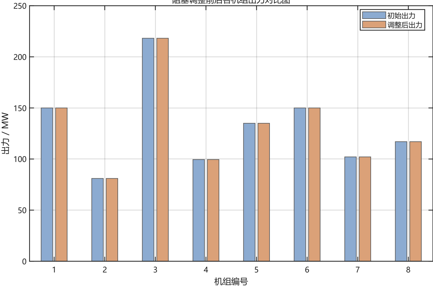
阻塞调整后各机组出力对比图
