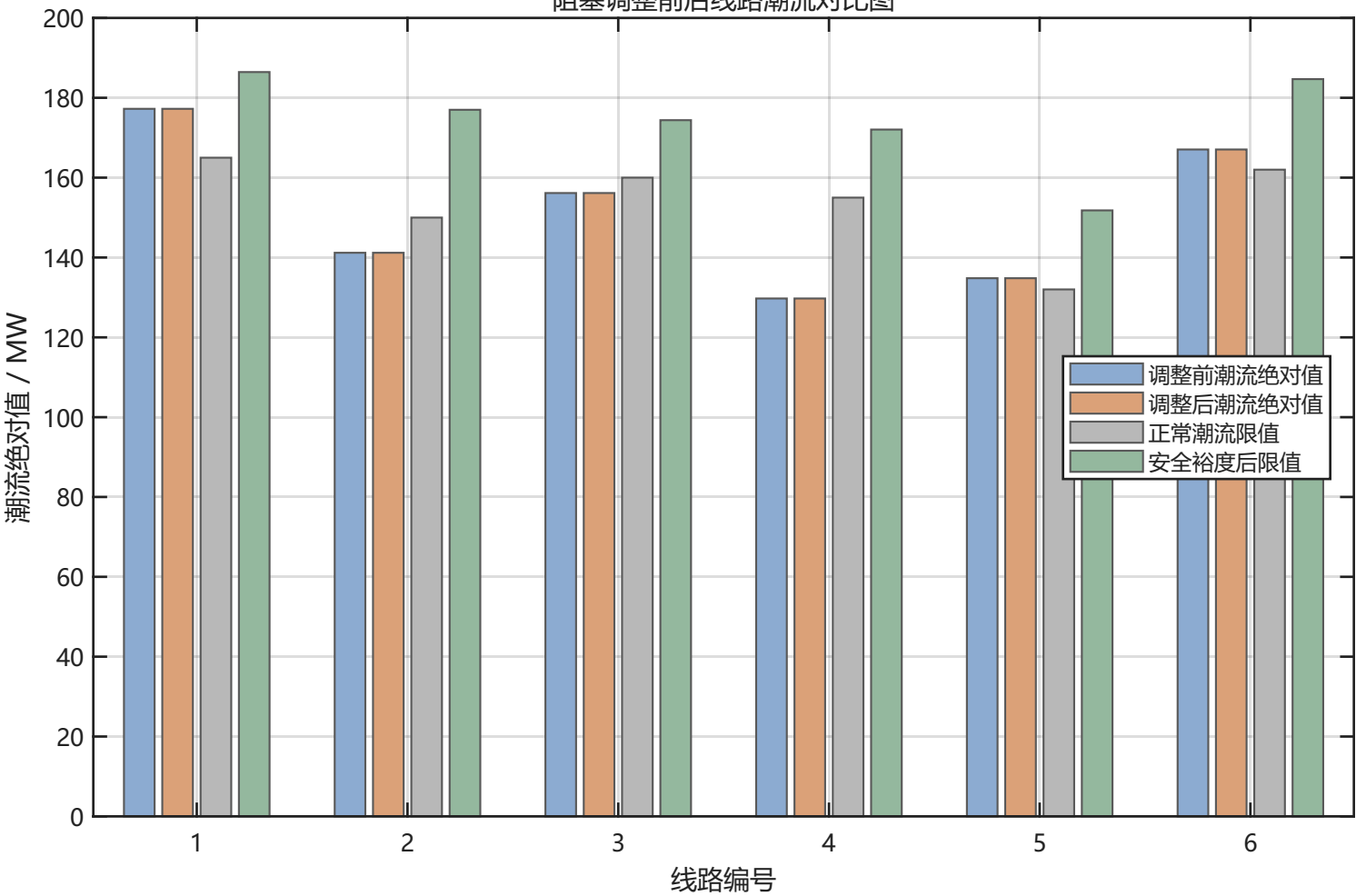
阻塞调整前后线路潮流对比图
