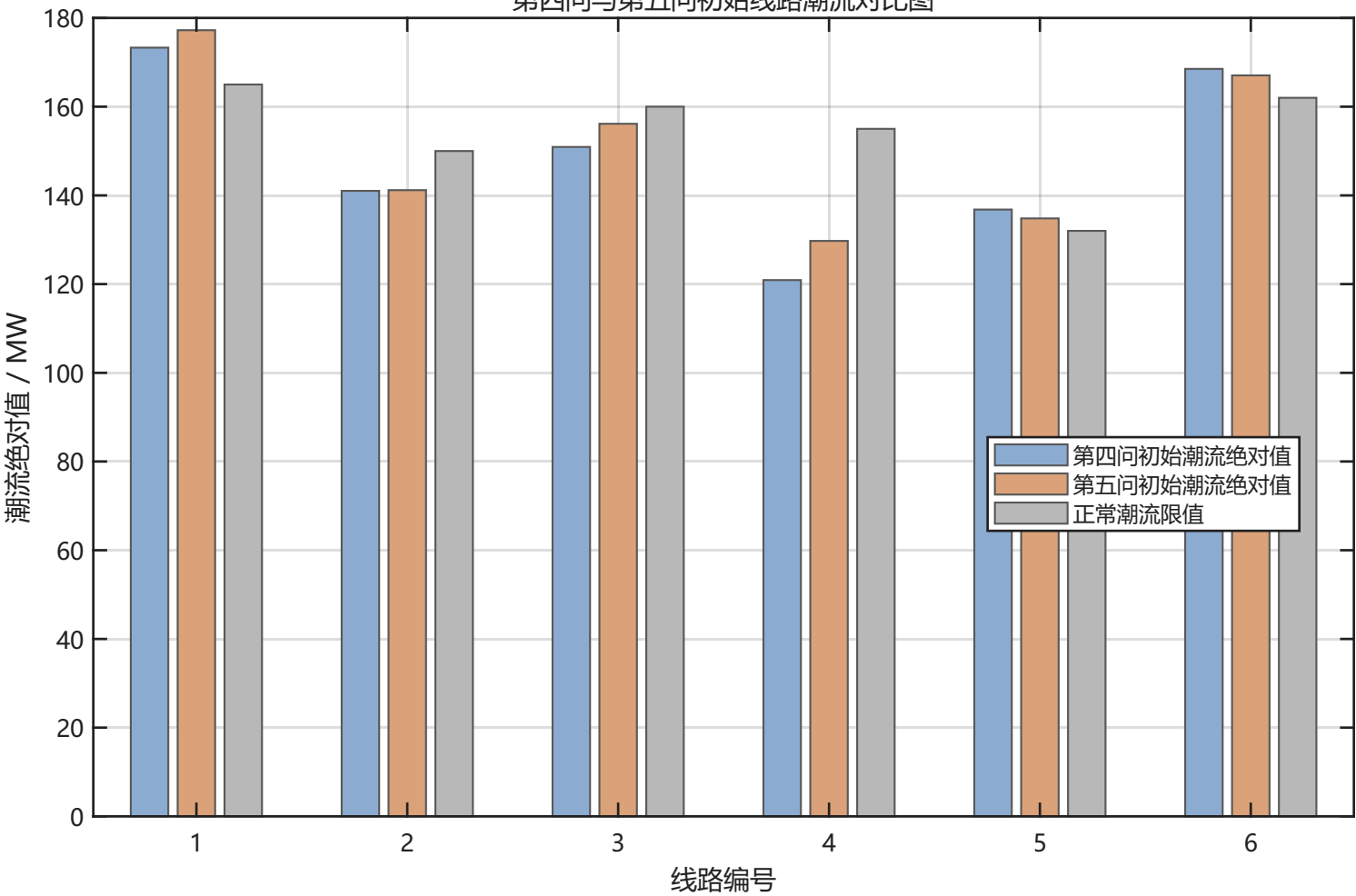
第四问与第五问初始线路潮流对比图
