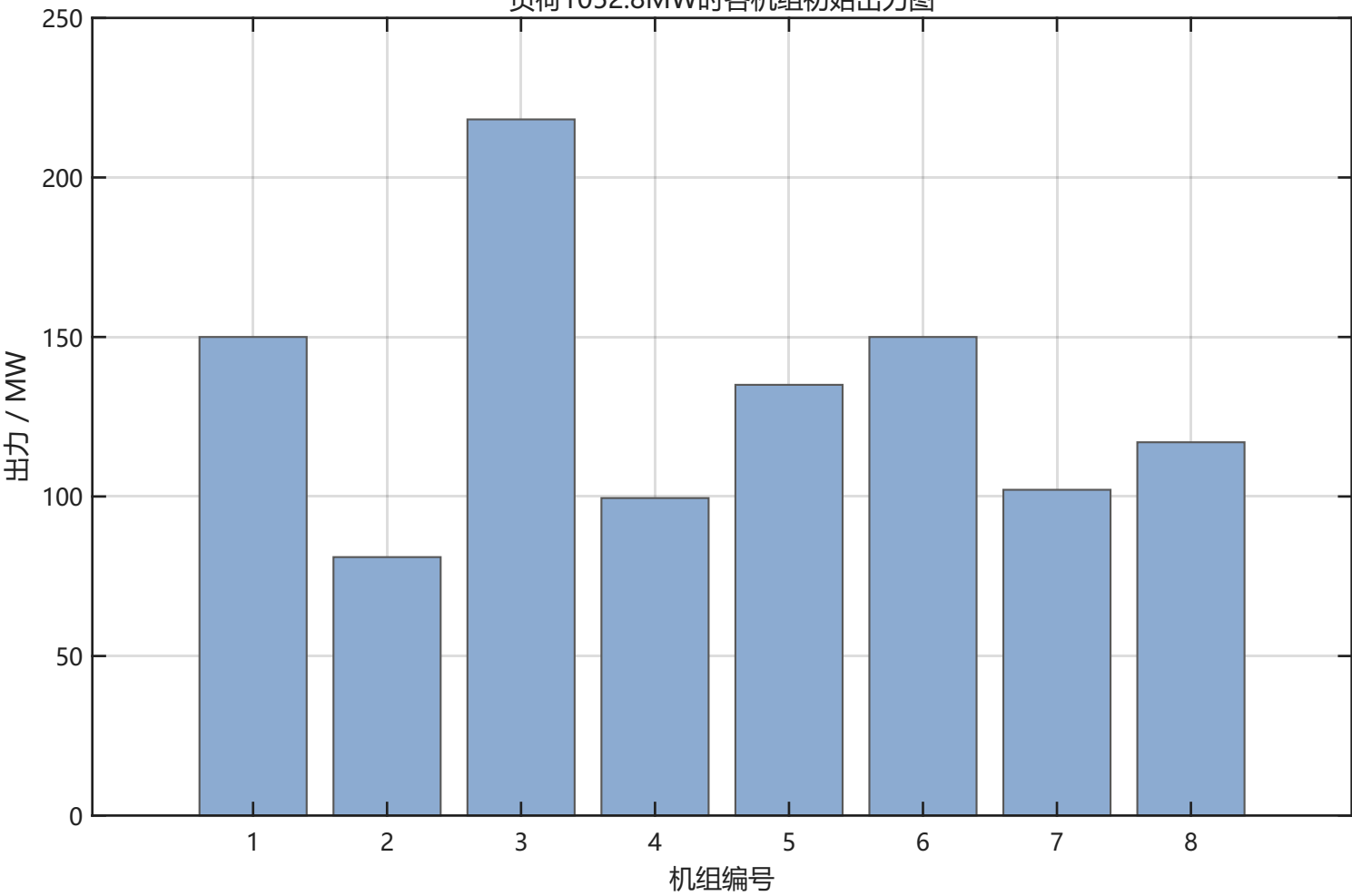
负荷1052.8MW时各机组初始出力图
