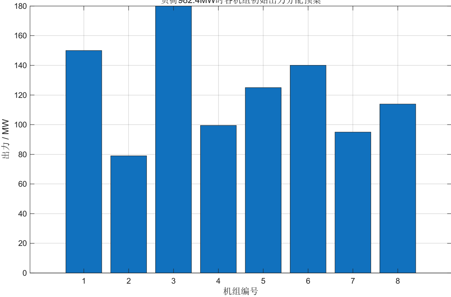
负荷982.4MW时各机组初始出力分配预案
