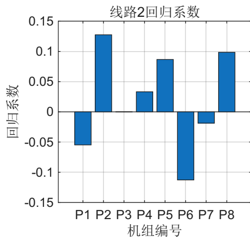
各线路潮流回归系数柱状图
