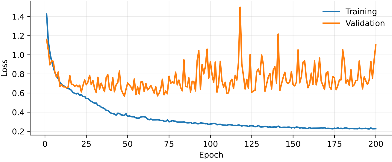
TCSF v3.1
