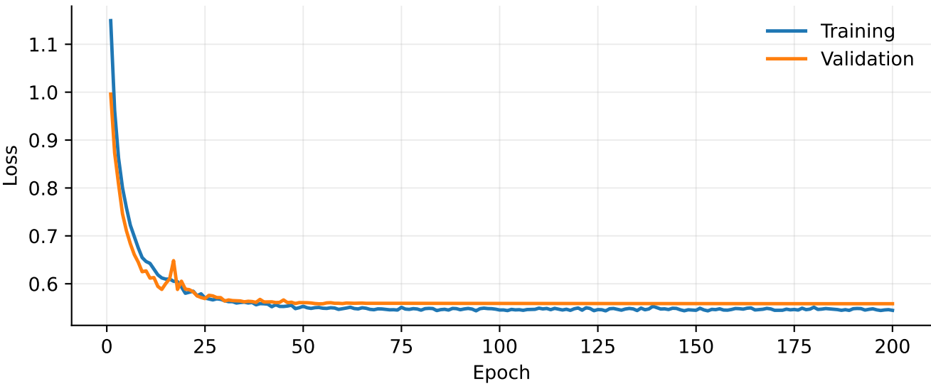
SegFormer-B0
