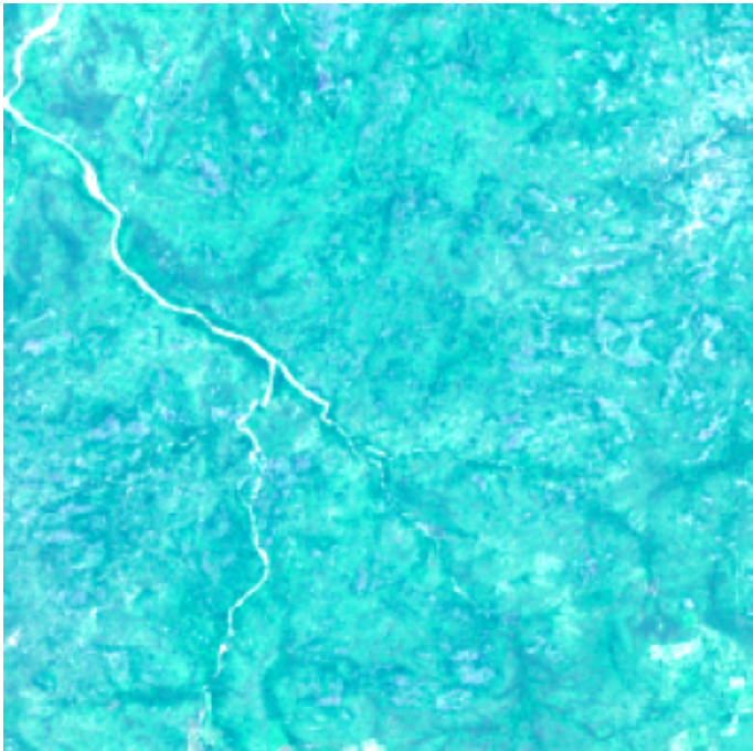
DeepLabV3+ IoU: 0.000
