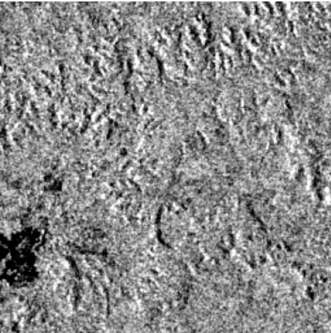
U-Net IoU: 0.573
