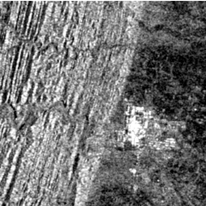
U-Net IoU: 0.000
