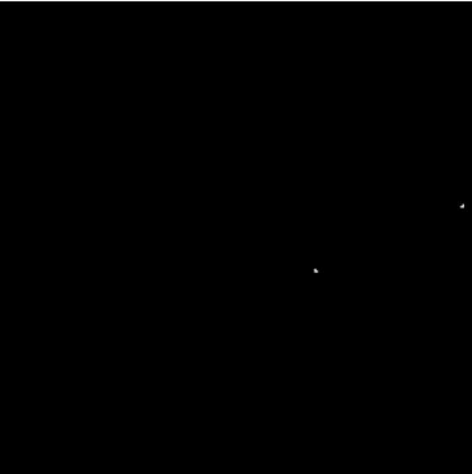
SegFormer-B0 IoU: 0.000
