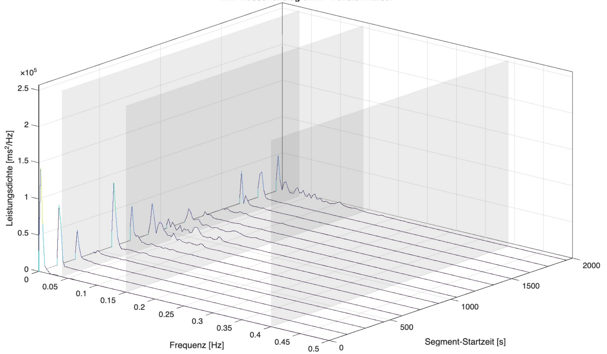
HRV-Wasserfalldiagramm - Fenster: kaiser
