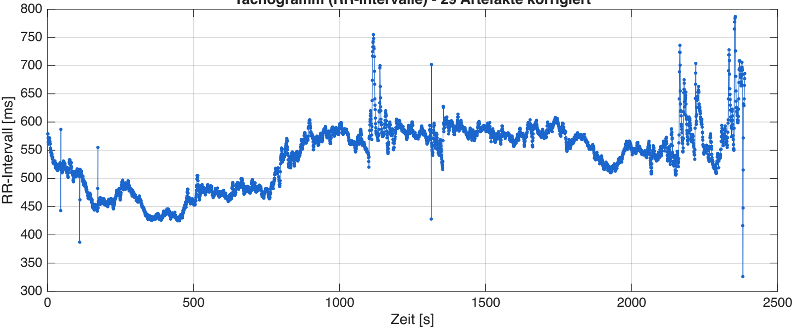
Tachogramm (RR-Intervalle) - 29 Artefakte korrigiert
