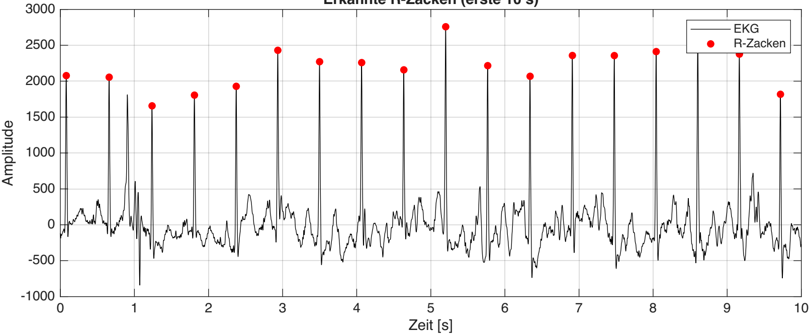
Erkannte R-Zacken (erste 10 s)
