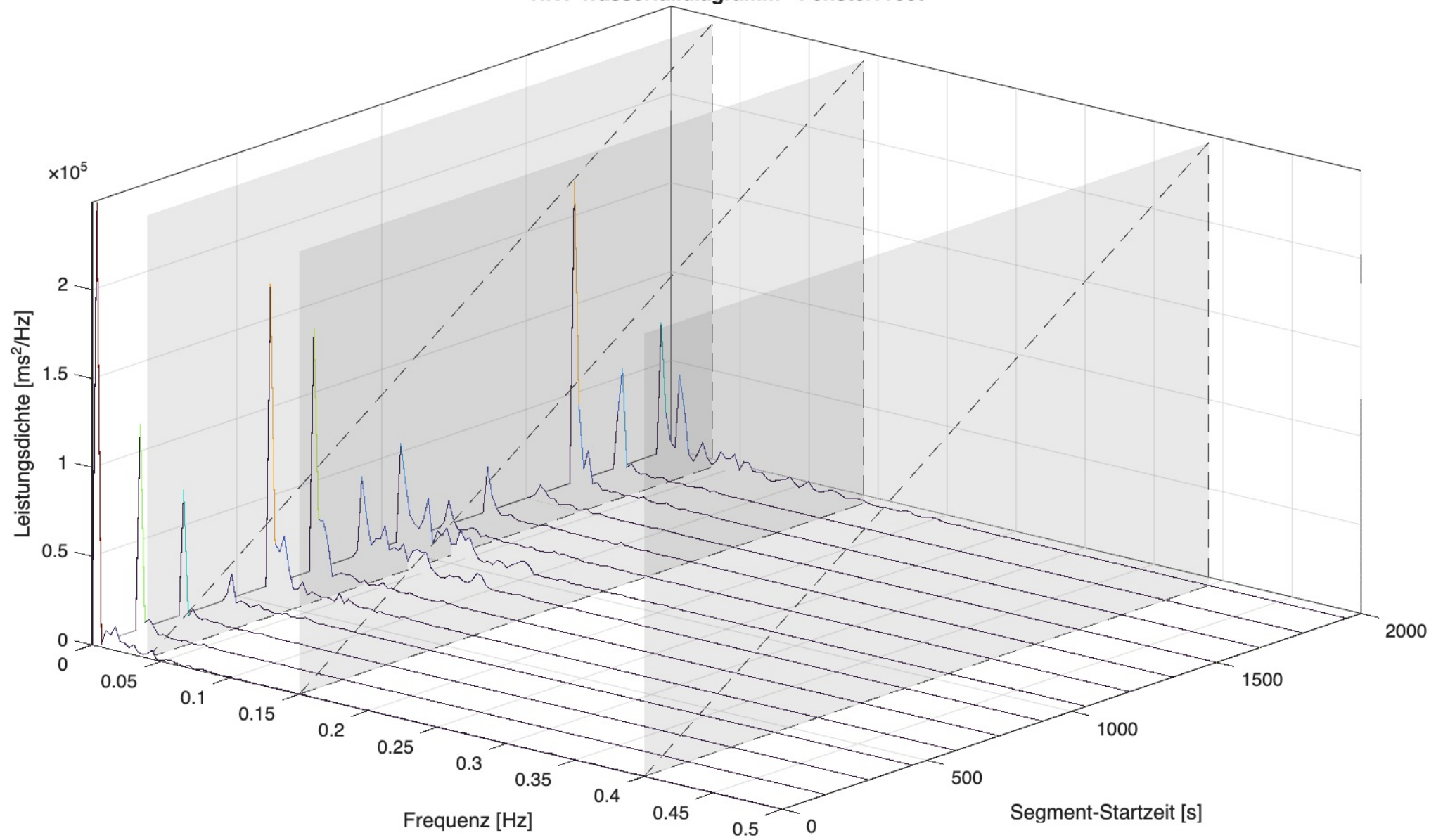
HRV-Wasserfalldiagramm - Fenster: rect
