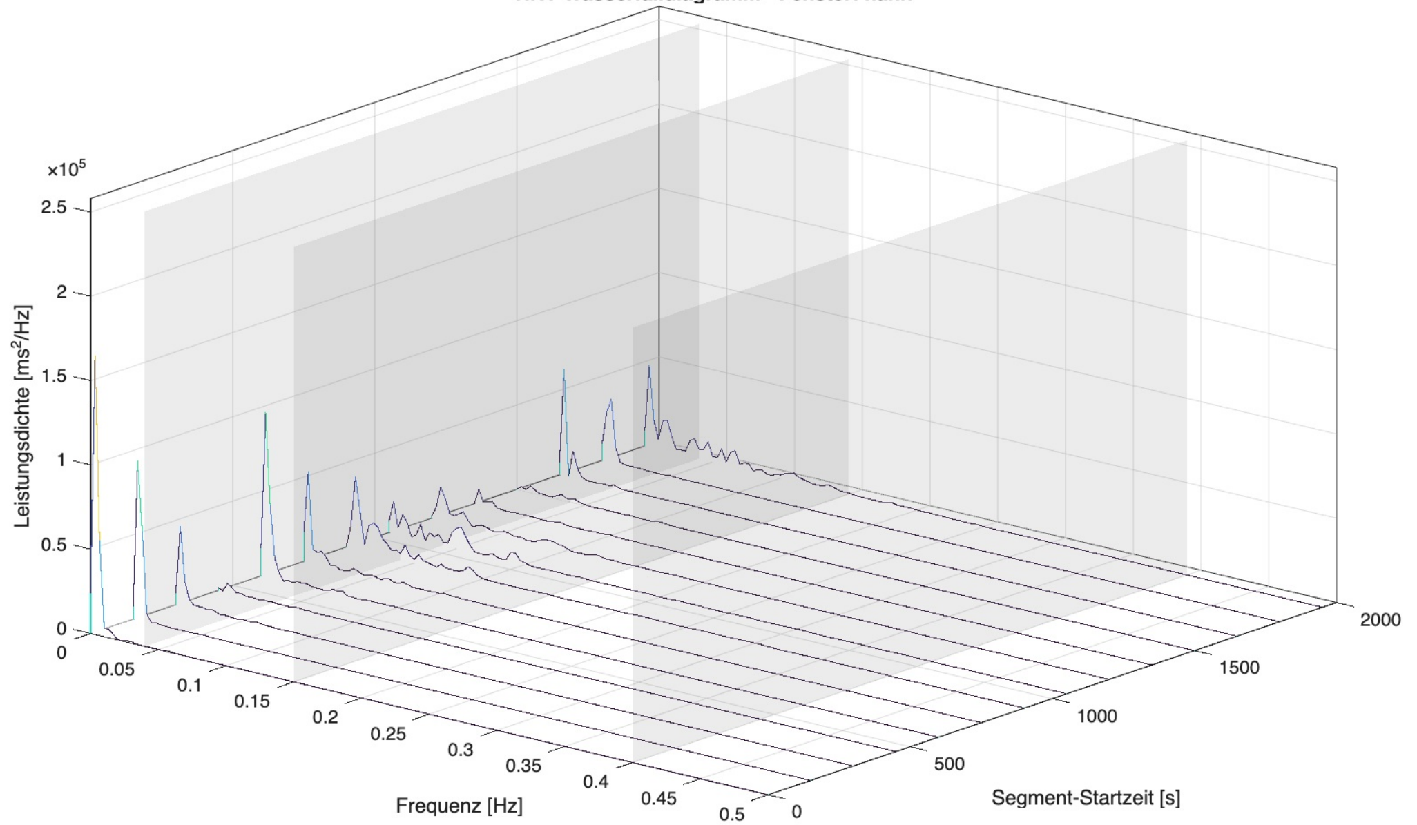
HRV-Wasserfalldiagramm - Fenster: hann
