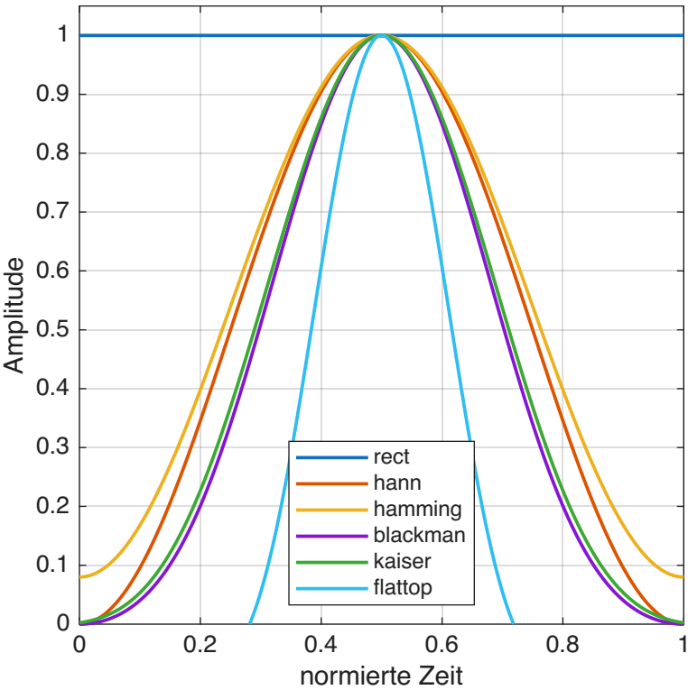
Fensterfunktionen - Zeitbereich
