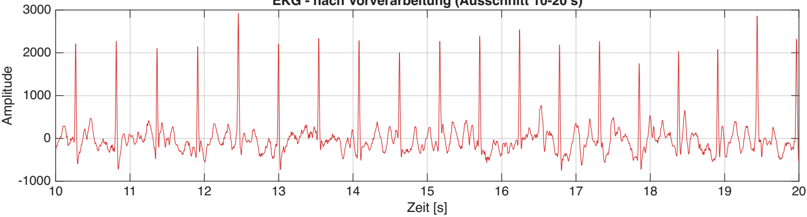
EKG - nach Vorverarbeitung (Ausschnitt 10-20 s)
