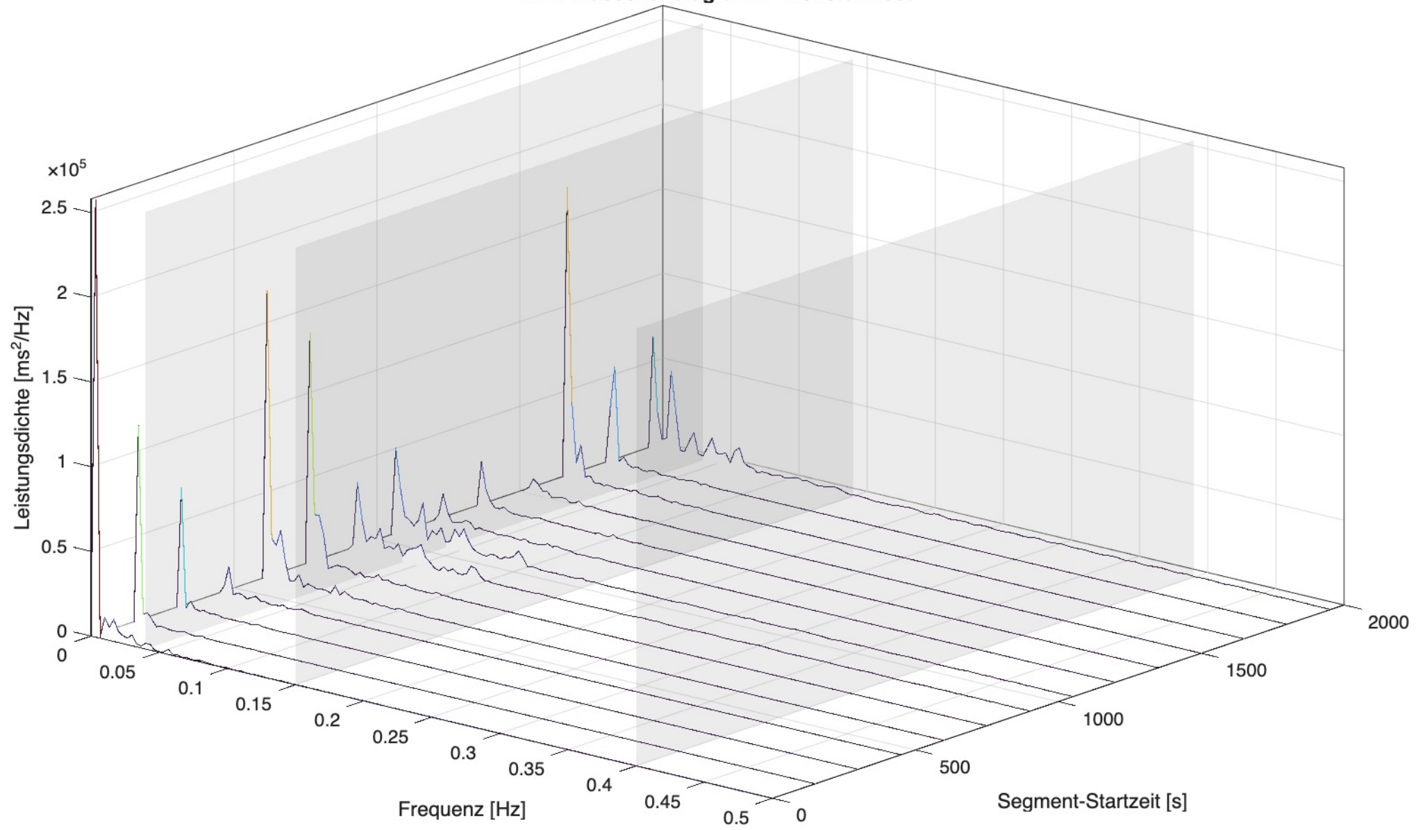
HRV-Wasserfalldiagramm - Fenster: rect
