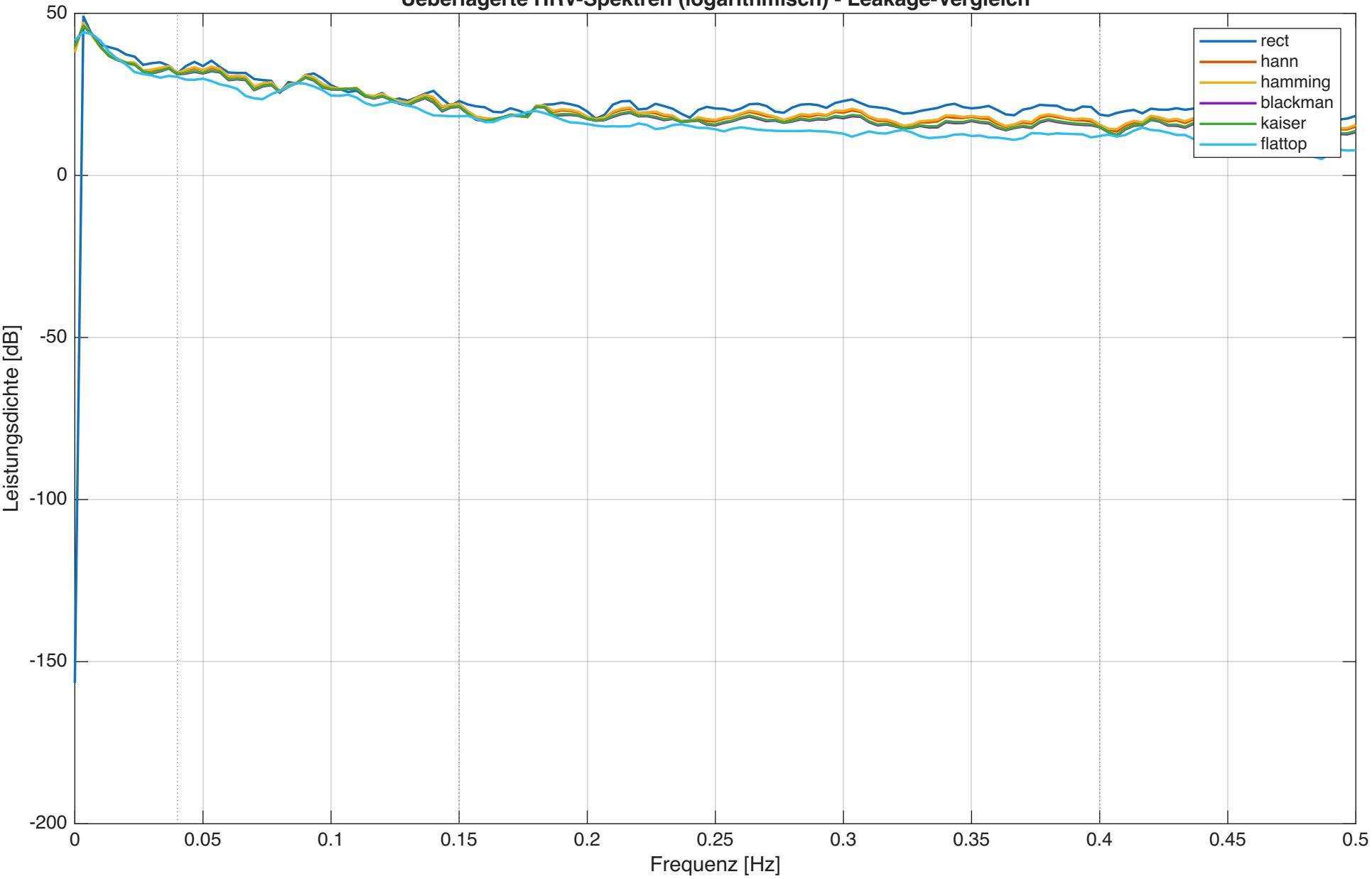
Ueberlagerte HRV-Spektren (logarithmisch) - Leakage-Vergleich
