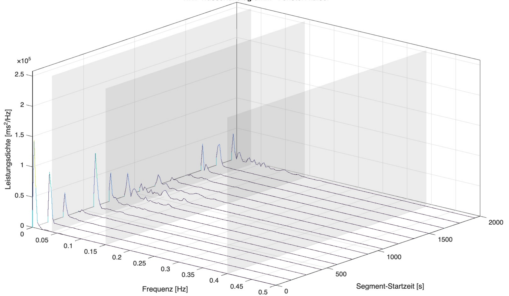
HRV-Wasserfalldiagramm - Fenster: kaiser
