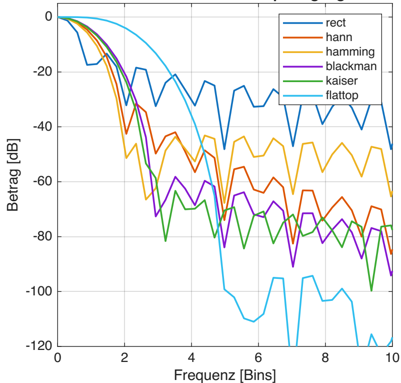
Fensterfunktionen - Frequenzgang
