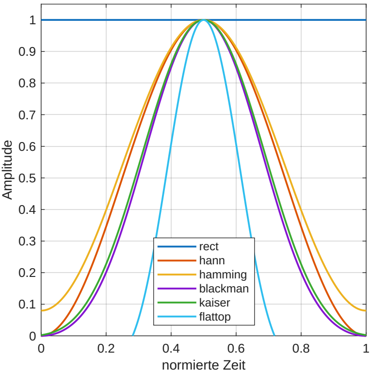
Fensterfunktionen - Zeitbereich
