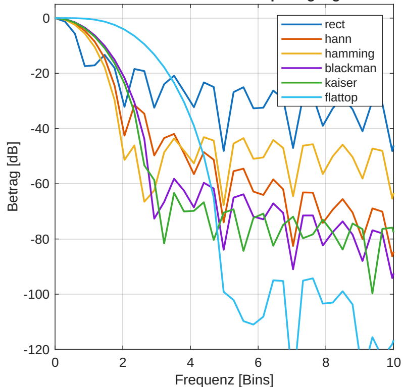
Fensterfunktionen - Frequenzgang
