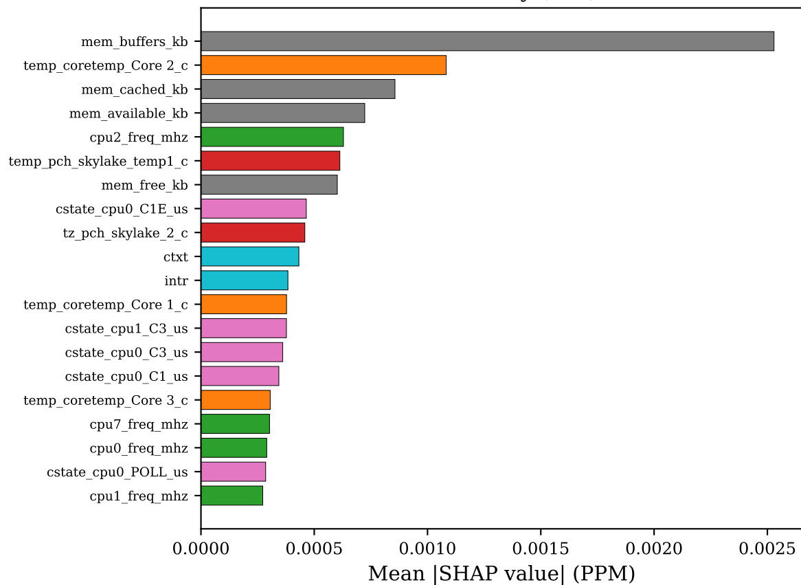
HPC (idle)
