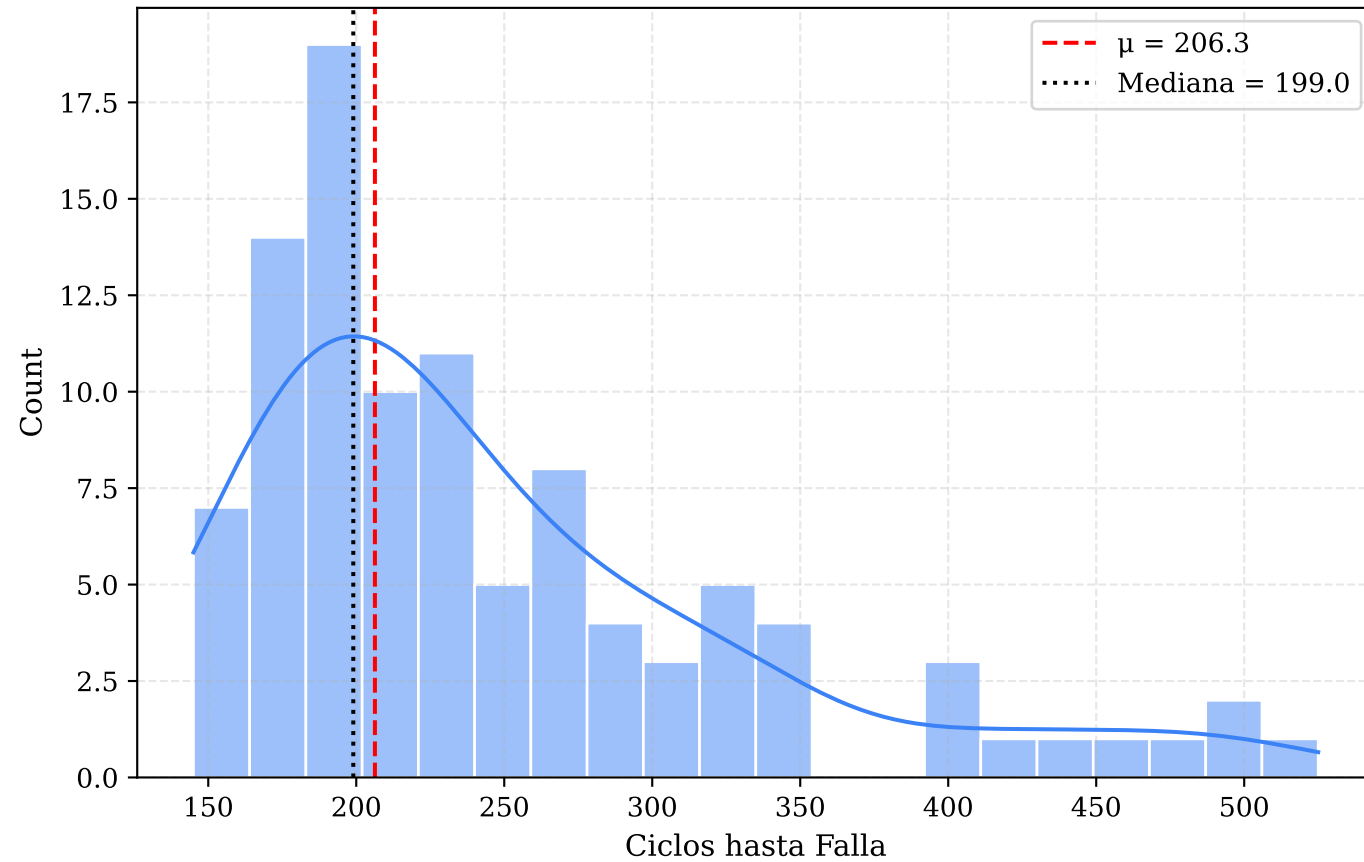
Distribución de Vida Útil (FD001 - 1 Modo de Falla)
