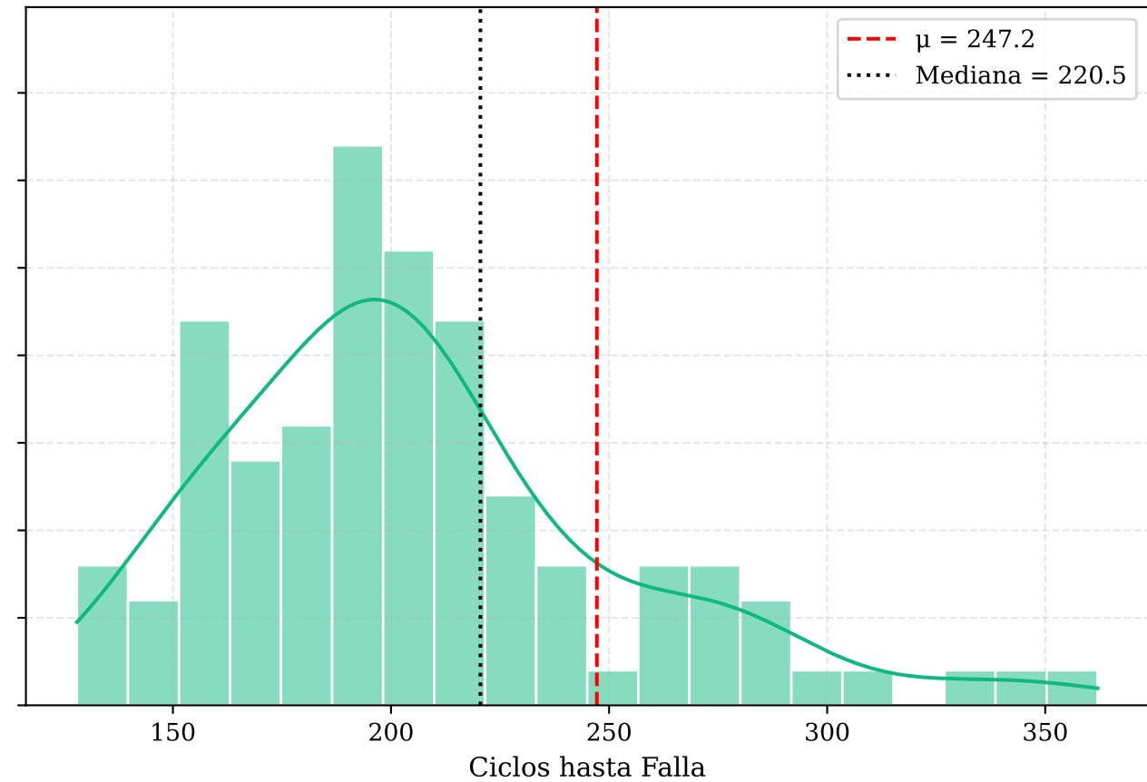
Distribución de Vida Útil (FD003 - 2 Modos de Falla)
