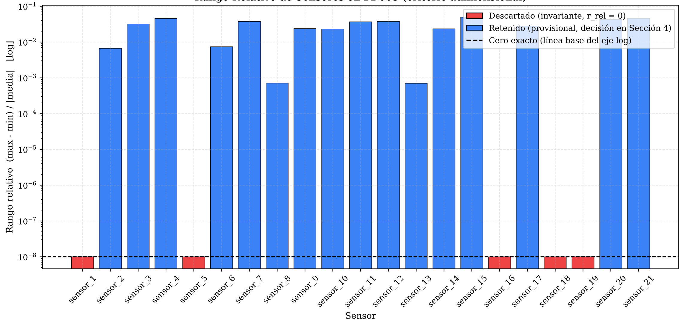
Rango Relativo de Sensores en FD003 (criterio adimensional)
