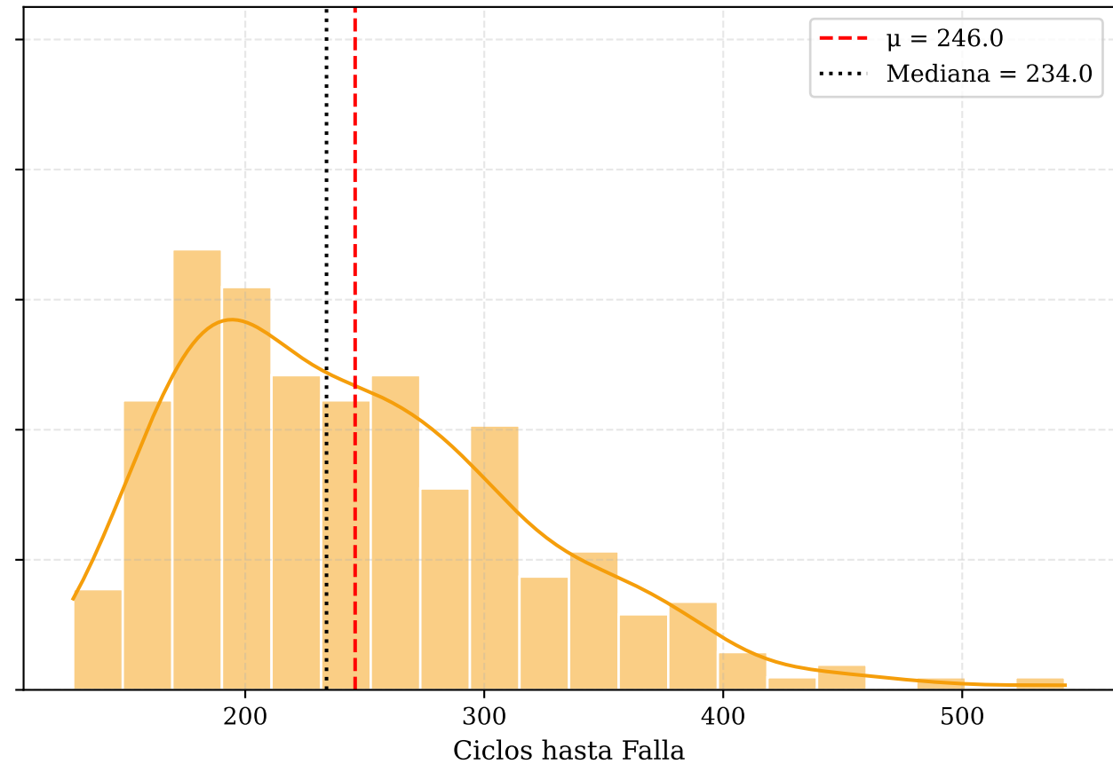
Distribución de Vida Útil (FD004 - 6 Regímenes, 2 Modos de Falla)
