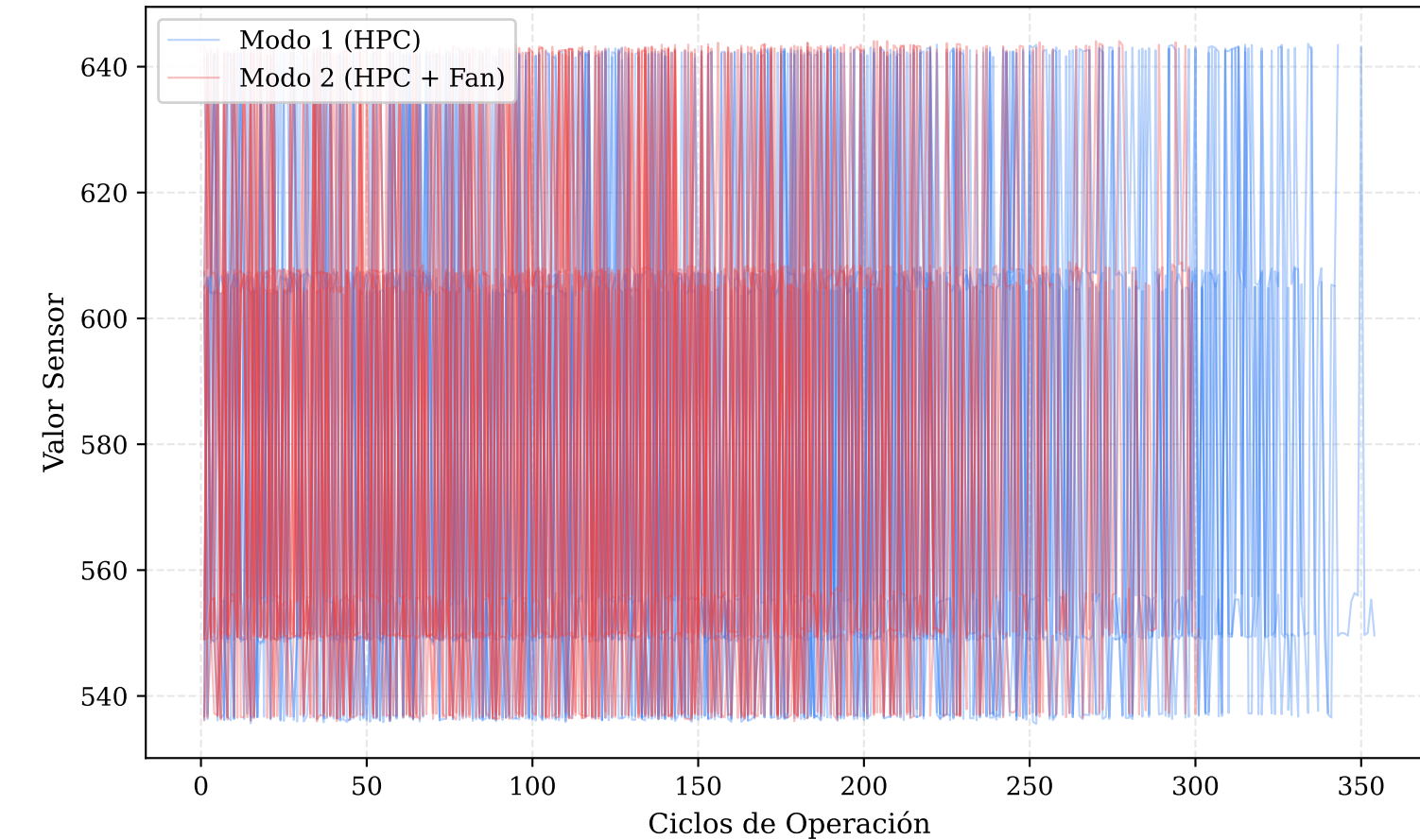
ESPACIO CRUDO (6 Regímenes Mixtos): sensor_2 (T24 - Salida LPC / Fan)
