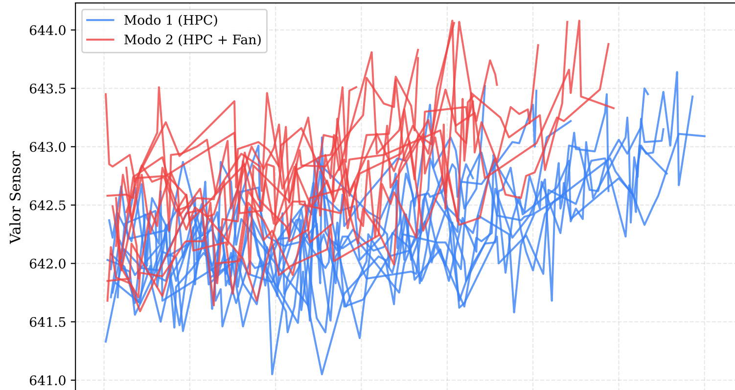
FÍSICA CONTROLADA (Régimen 4): sensor_2 (T24 - Salida LPC / Fan)
