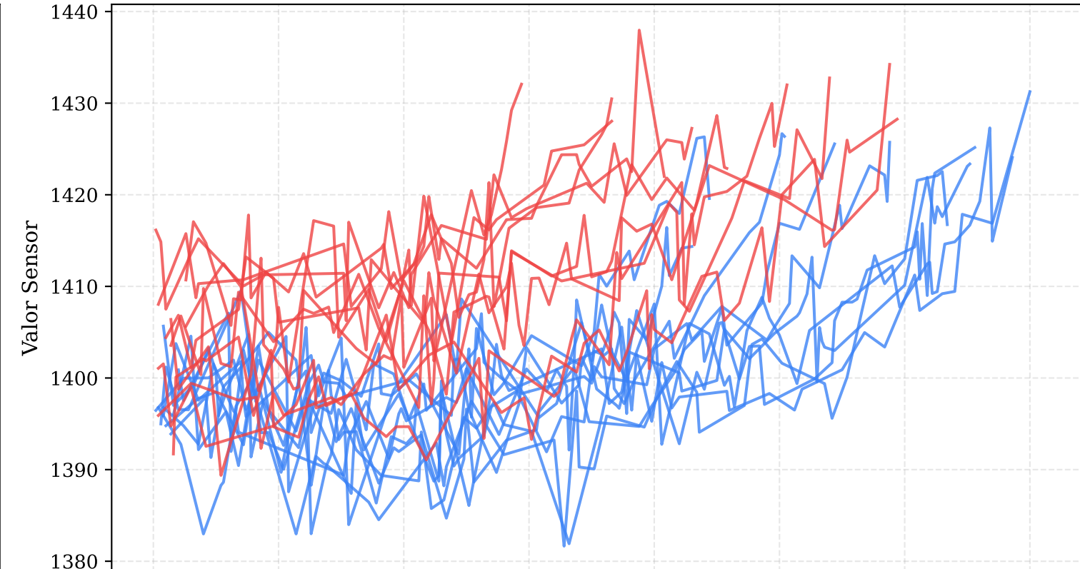
FÍSICA CONTROLADA (Régimen 4): sensor_4 (T50 - Salida LPT)
