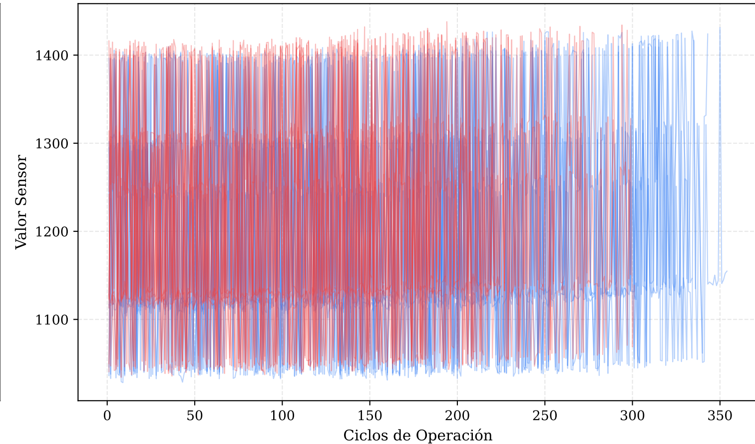
ESPACIO CRUDO (6 Regímenes Mixtos): sensor_4 (T50 - Salida LPT)
