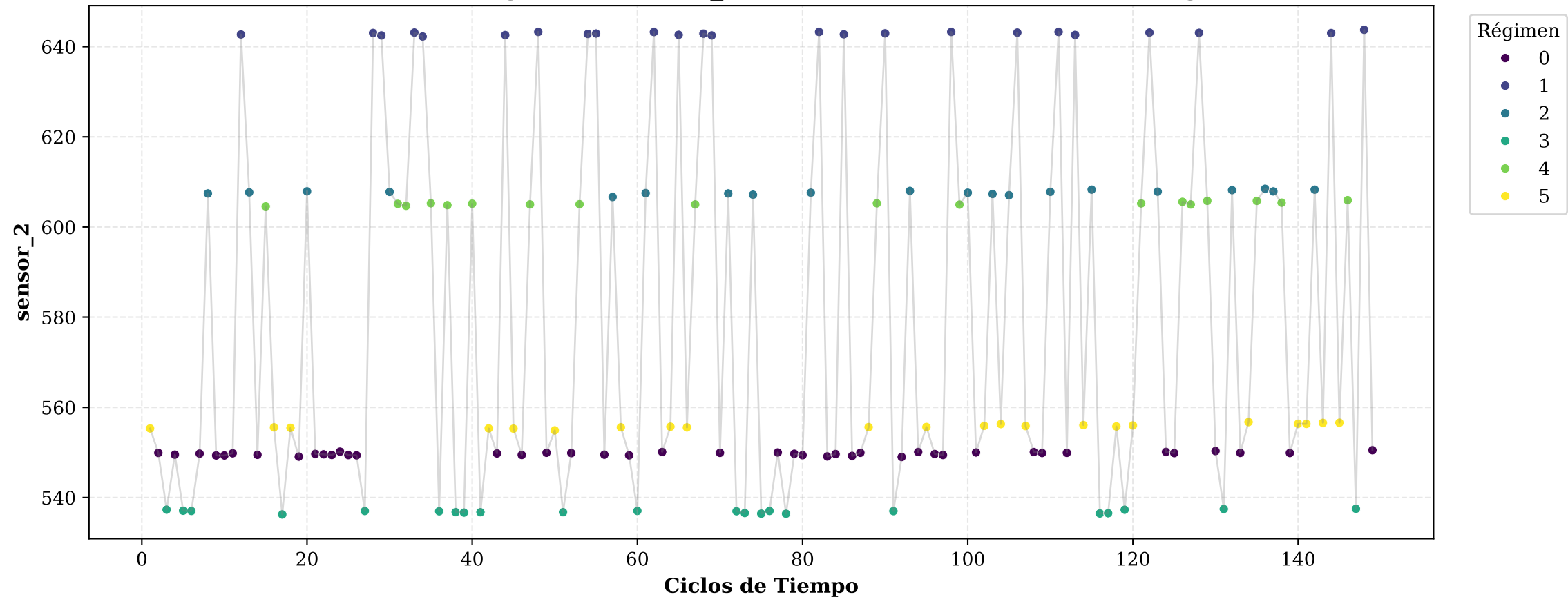
Evolución Cronológica de sensor_2 en Motor 1 (Coloreado por Régimen)
