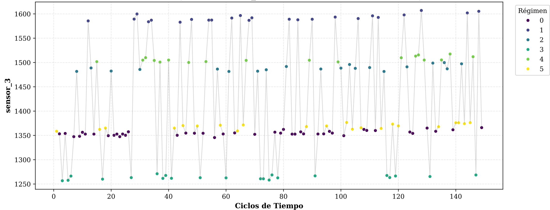
Evolución Cronológica de sensor_3 en Motor 1 (Coloreado por Régimen)
