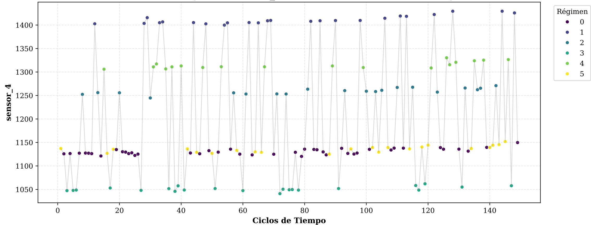
Evolución Cronológica de sensor_4 en Motor 1 (Coloreado por Régimen)
