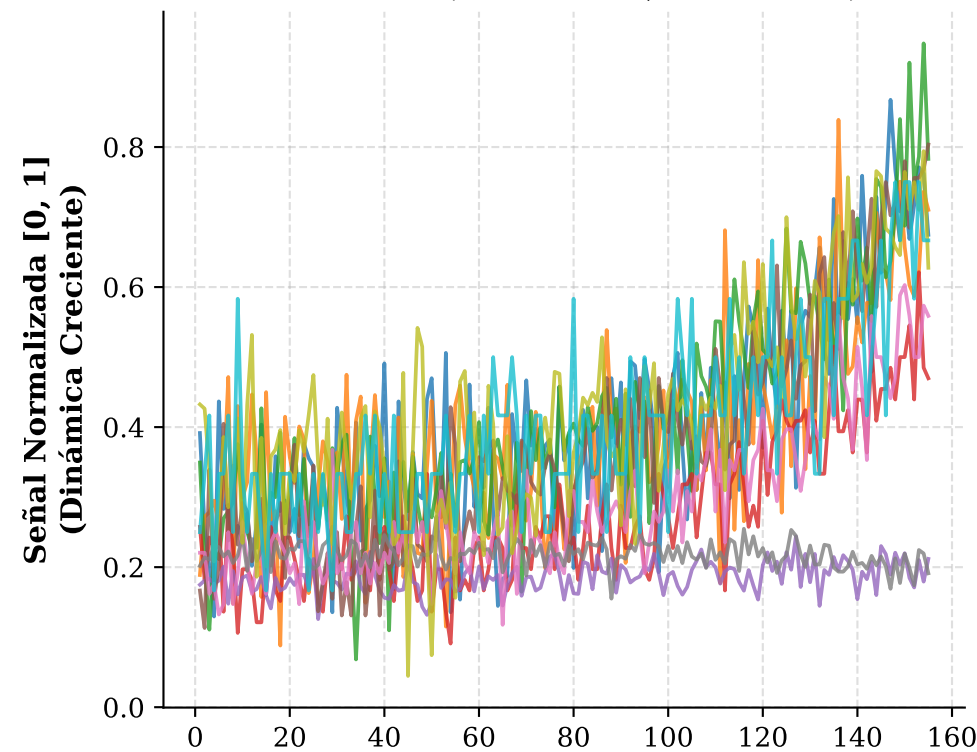
Motor 93 (Vida Corta, 155 ciclos)
