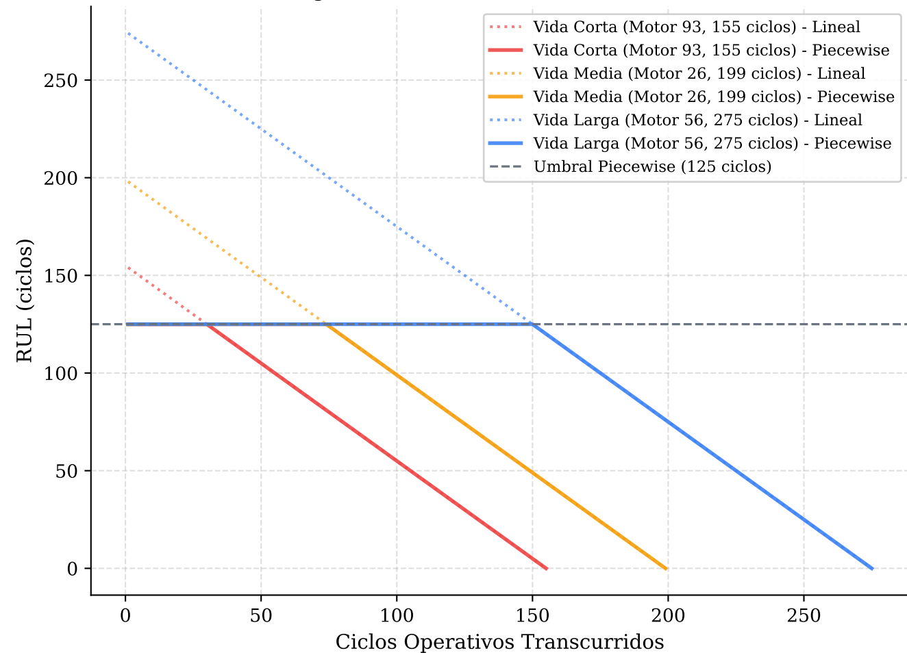
Perfil Objetivo: RUL Lineal vs. Piecewise RUL
