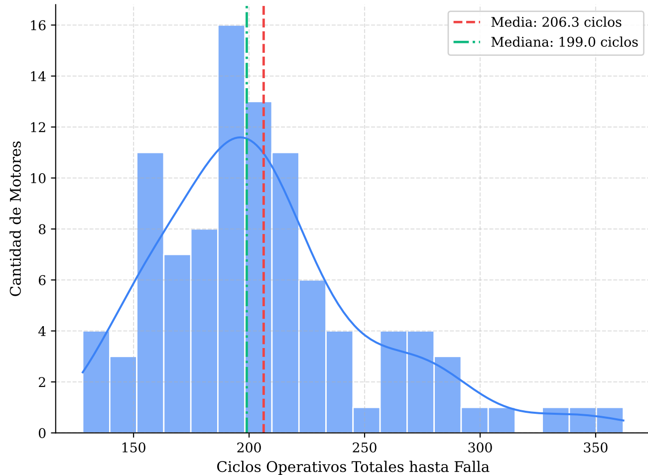
Distribución de Vida Útil Total de Motores (FD001)
