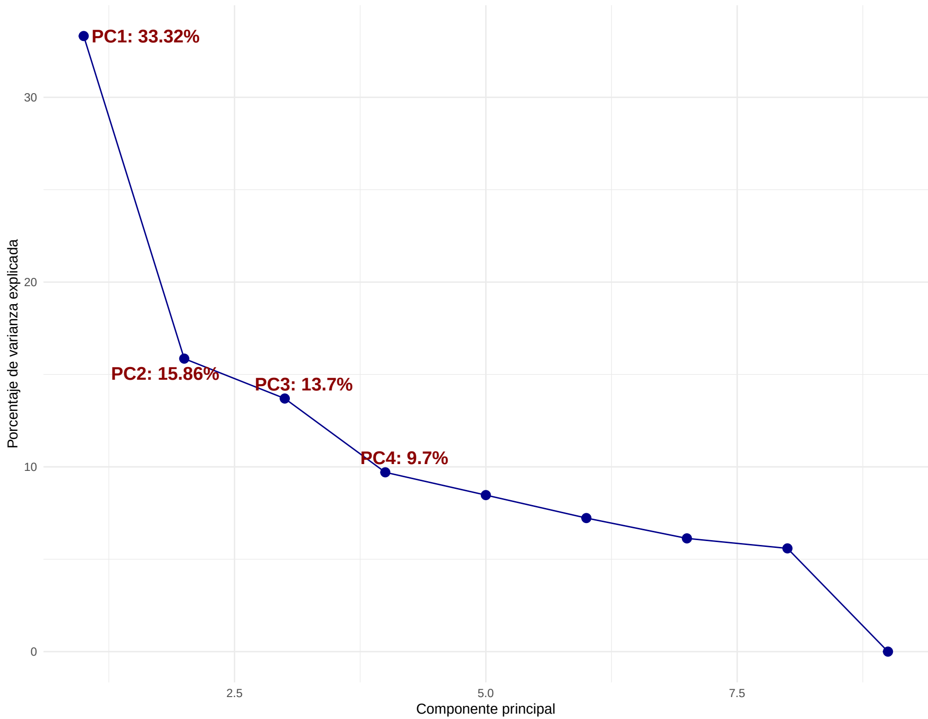
Scree plot: varianza explicada por PCA
